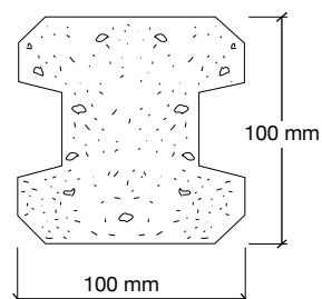
Profil af betonstolpe
