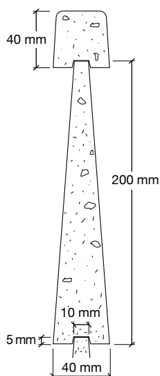
Profil af plade + top
